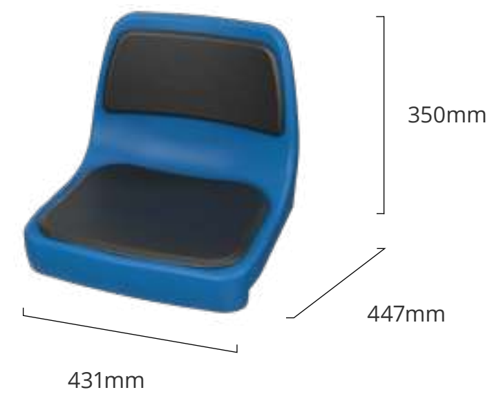
Stadion-/tribunestoel CR-4 (met polster)
