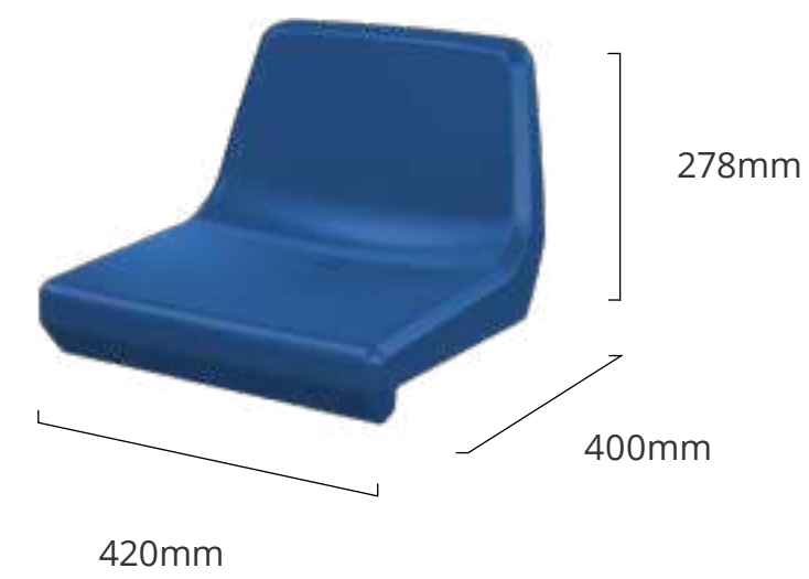
Stadion-/tribunestoel CR-3
